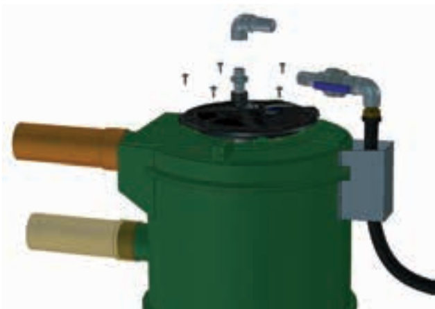
3. Montera pumpen. Notera att pumpen skall monteras vriden så att utloppsrörets position ligger klockan 2 om inloppen ligger klockan 12.
