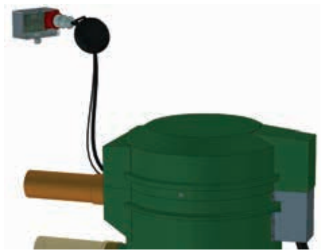
6. Provkör och testa larmfunktionen enligt checklistan på följande sidor. Sätt på skyddslocket och fäst detta med de två skruvarna.
